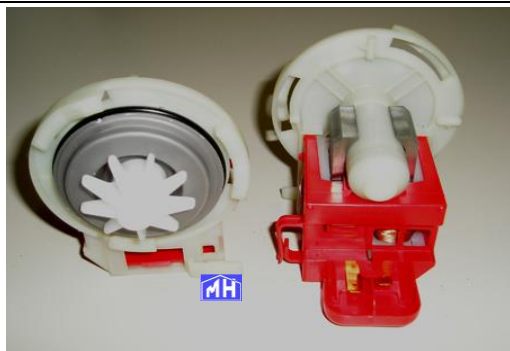
LV160501 - BOMBA LVV. BALAY BAYONETA COPRECI
