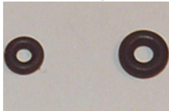
JUNTA TAPA MEMBRANA Y CASQUILLO CALENTADOR COINTRA CA272001 - Ø ext. 4,8 mm. grosor 1,5 mm. (para CA271101 y CA271102) CA272002 - Ø ext. 7,6 mm. grosor 1,8 mm. (para CA271104)
